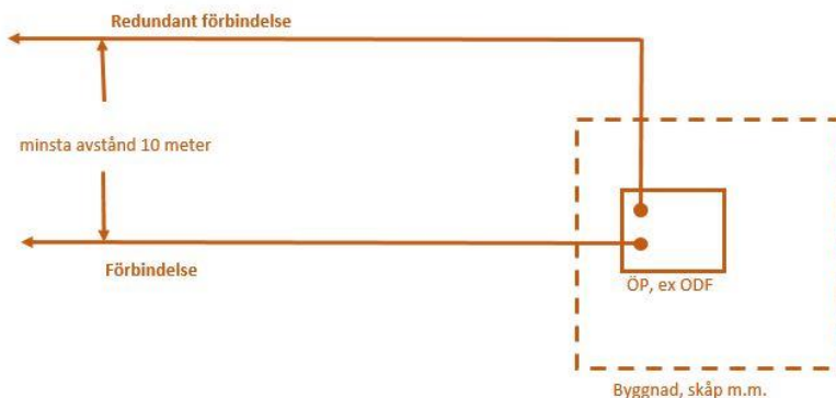
Bild: Exempel: Redundans utan markbrunn
